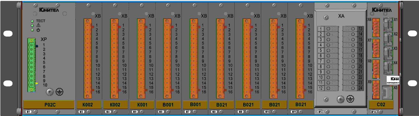
Рисунок 1.1 – Вид устройства «ЮНИТ-М319-Т» с размещением модулей по слотам (исполнение для I архитектуры)
