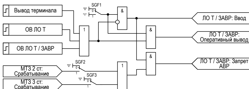
Рисунок 2.23 – Функциональная схема «ЗАВР»
