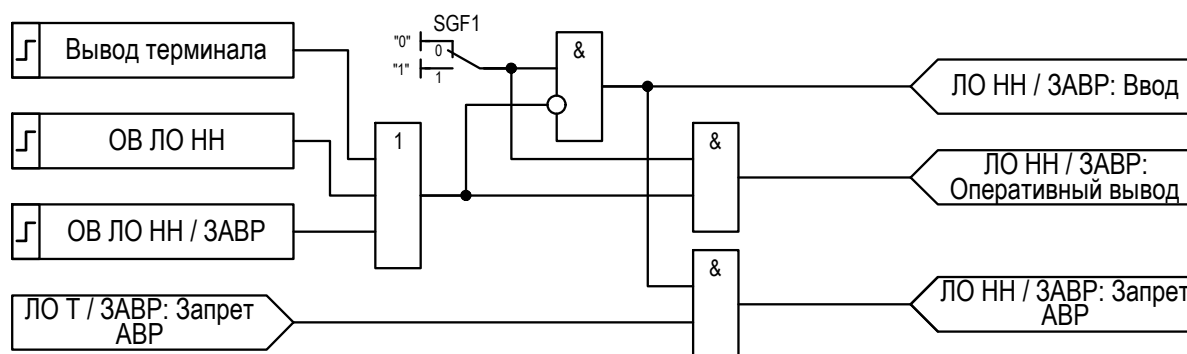
Рисунок 2.27 – Функциональная схема «Запрет АВР»
